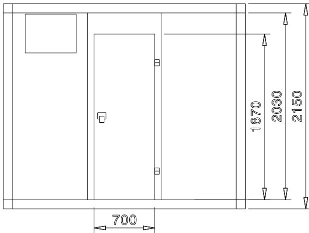
Zij aanzicht
